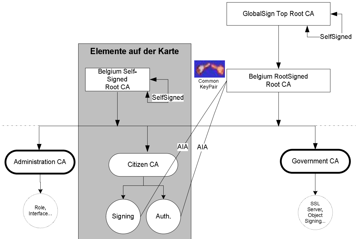
Abbildung 1: eID-Hierarchie
