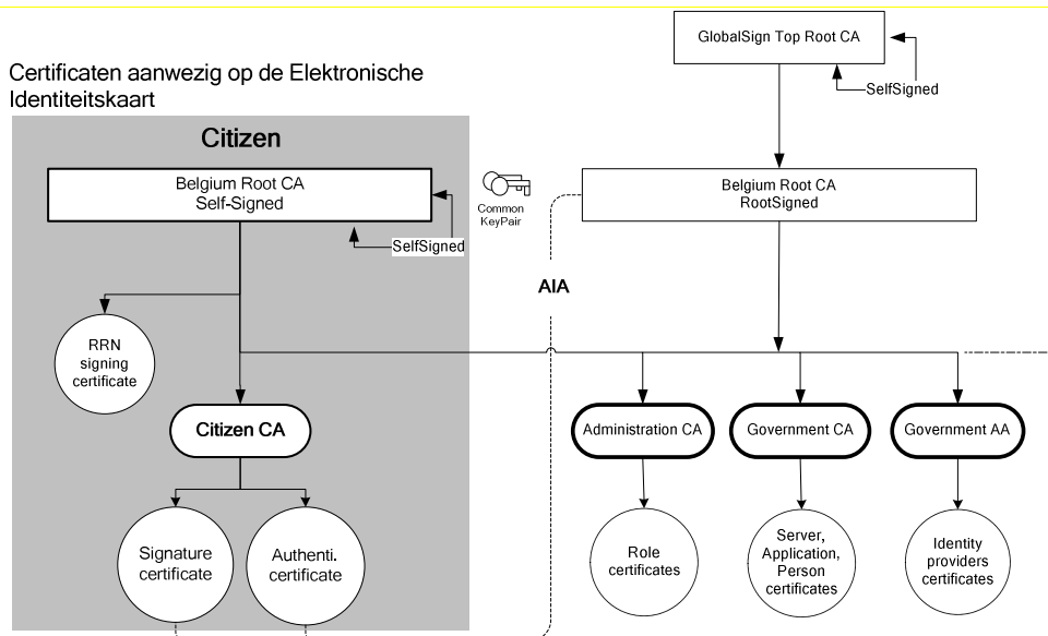
Figuur 1: PKI-hiërarchie
